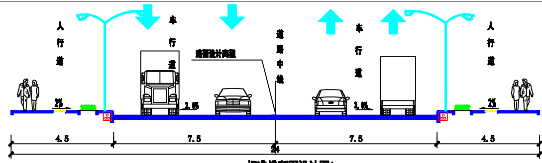
标准横断面设计图1 K0+000~K0+219.47
