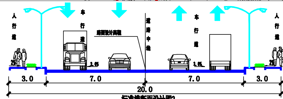
标准横断面设计图2 K0+219.47~K0+695.325
