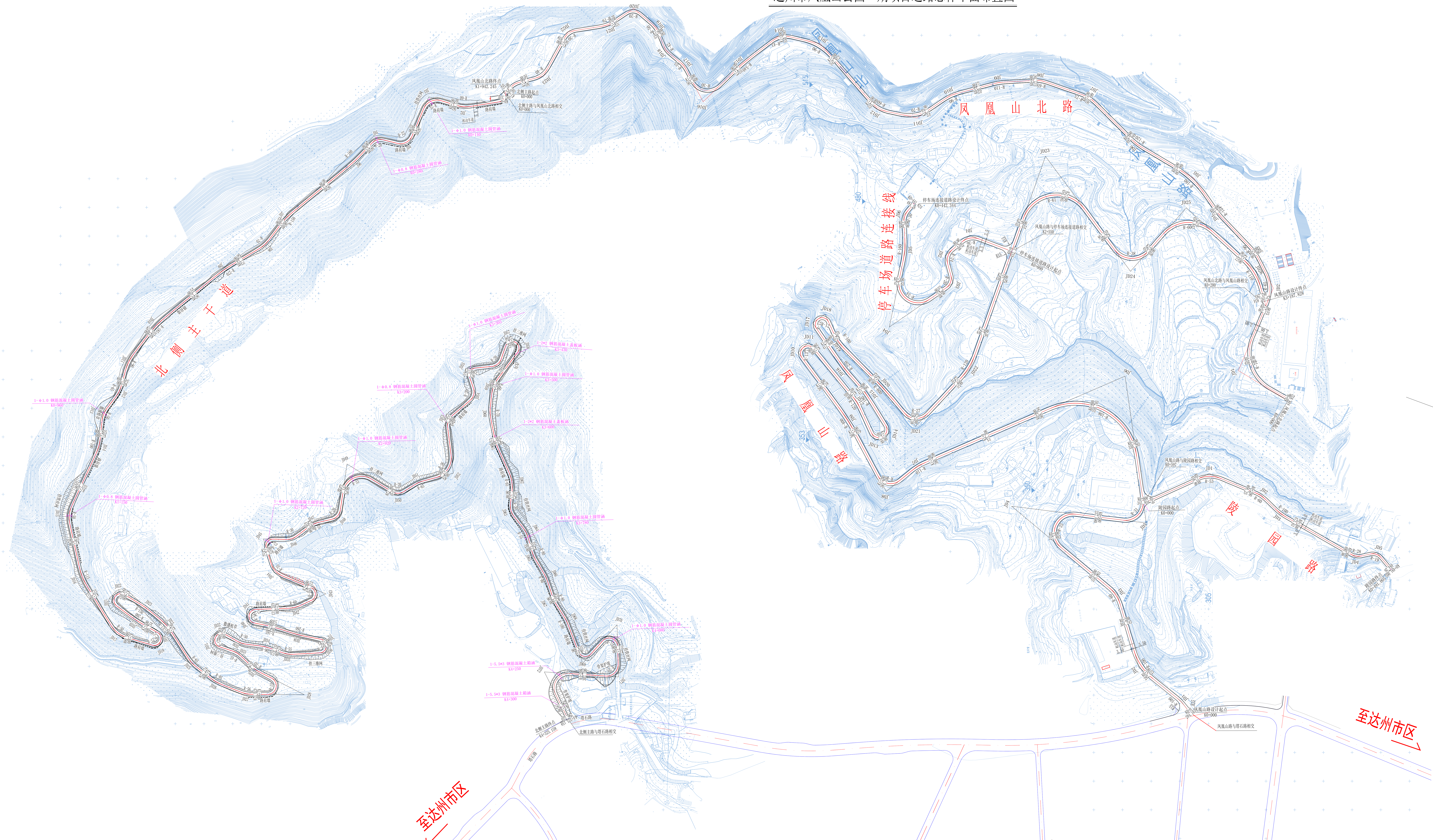
达州市凤凰山公园一期项目道路总体平面布置图
