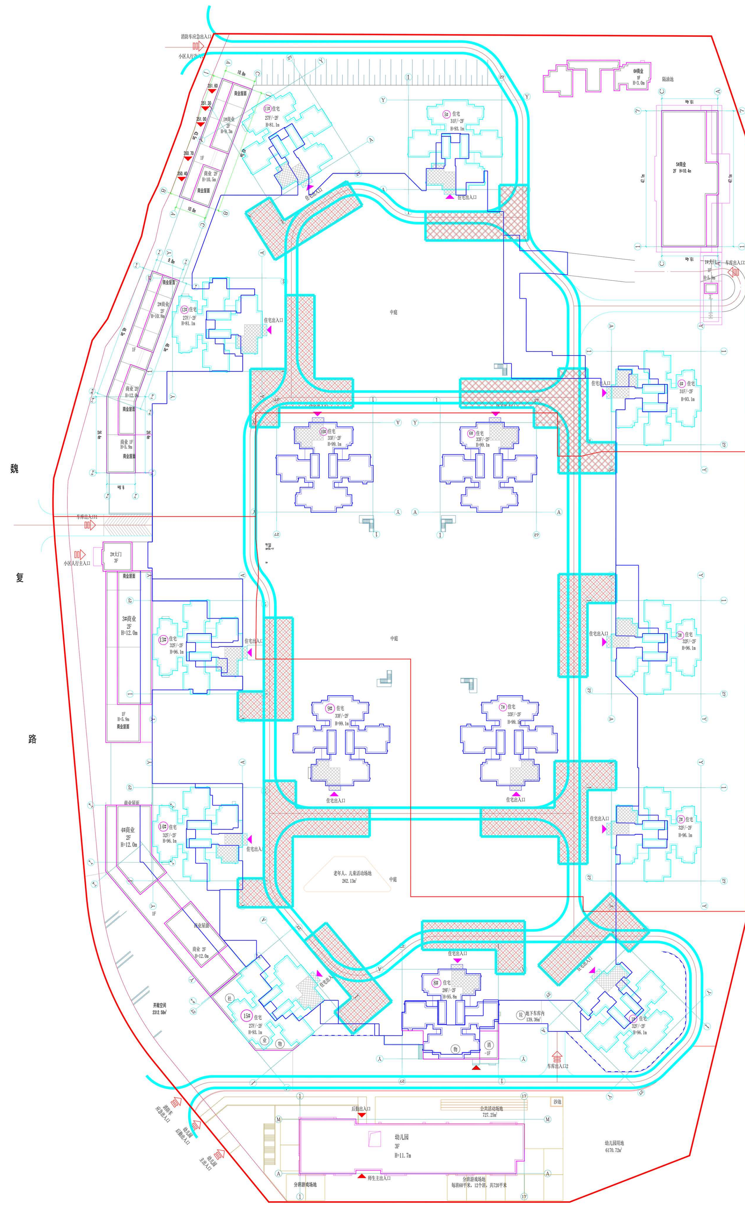
规划审批项目平面图
